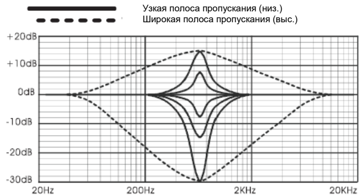
Параметрический эквалайзер
